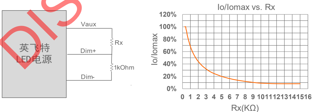
示意图 3: 电阻曲线
