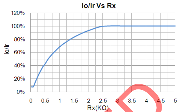
示意图 2 : 电阻曲线
