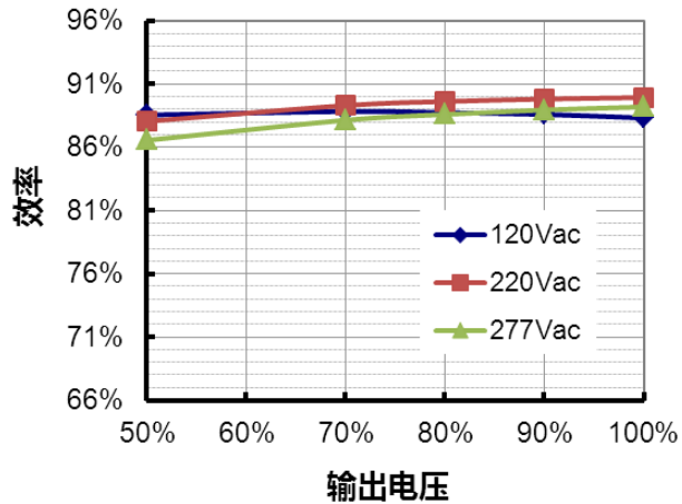
EUC-052S045DT(ST) 效率 vs. 输出电压
